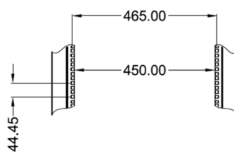
Dimensión de montaje
