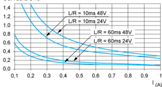
Curvas DC13
