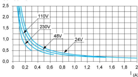
Curvas AC14
